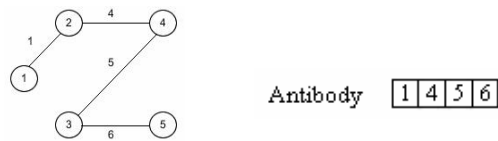
Fig. 3. Codification example
