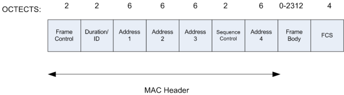
Fig. 2. MAC frame format [5]
